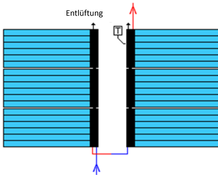
Anschlussschema DF6 Fassade 2-8 Module in Reihe
