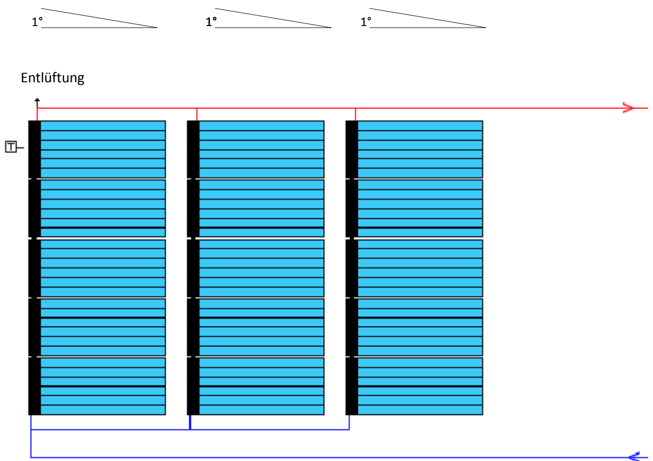
Anschlusschema DF6 Fassade für gleichgroße Felder ab 8 Modulen
